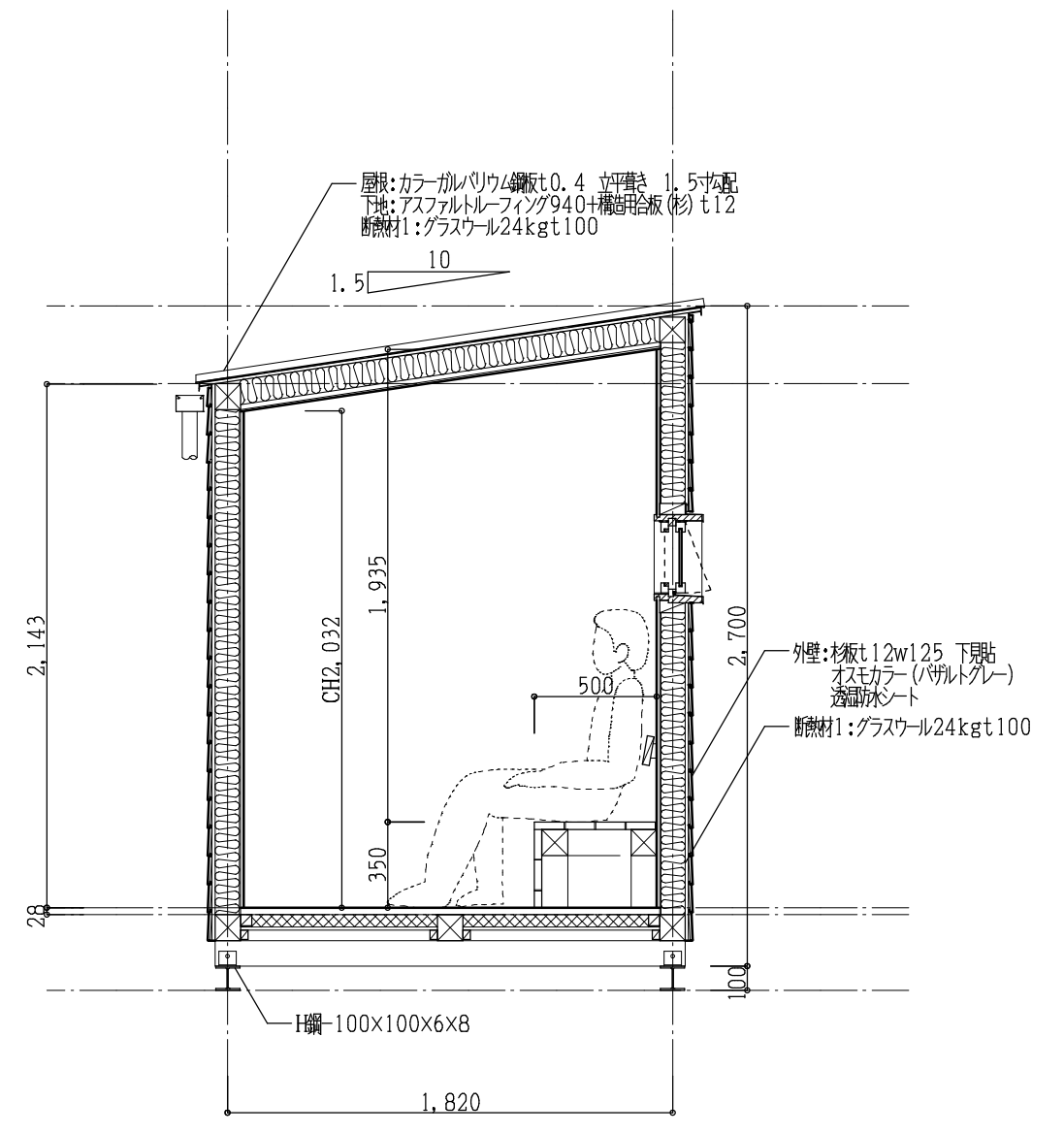
矩計図 S: 1/30
